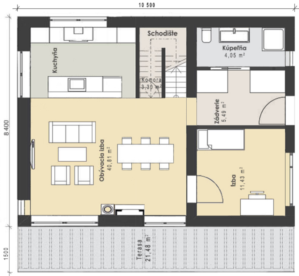
PÔDORYS 1.NP
